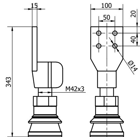
Isolator DN / LV bushing / US-Durchführungen / Raccordement BT
