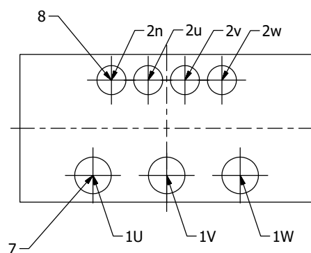
Zaciski / Terminals / Klemmen / Terminaux
