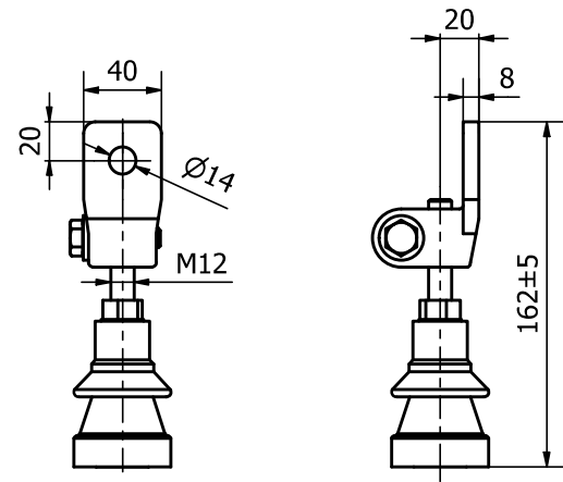
Izolator DN / LV bushing / US-Durchführungen / Raccordement BT
