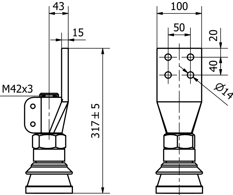
Izolator DN / LV bushing / US-Durchführungen / Raccordement BT
